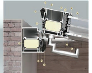
Cửa đi DW70 có cầu cách nhiệt
